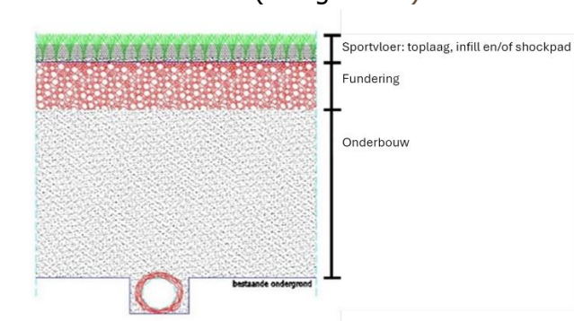
Figuur 2.1 Opbouw van een kunstgras sportveld
