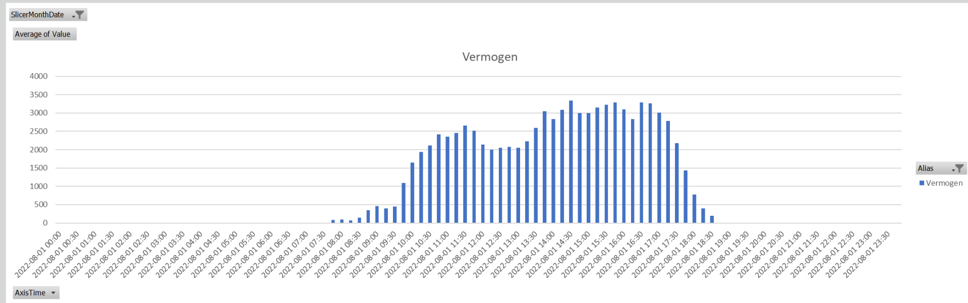
Figuur 2: vermogen gemeten op 1-augustus-2022 in Watt
