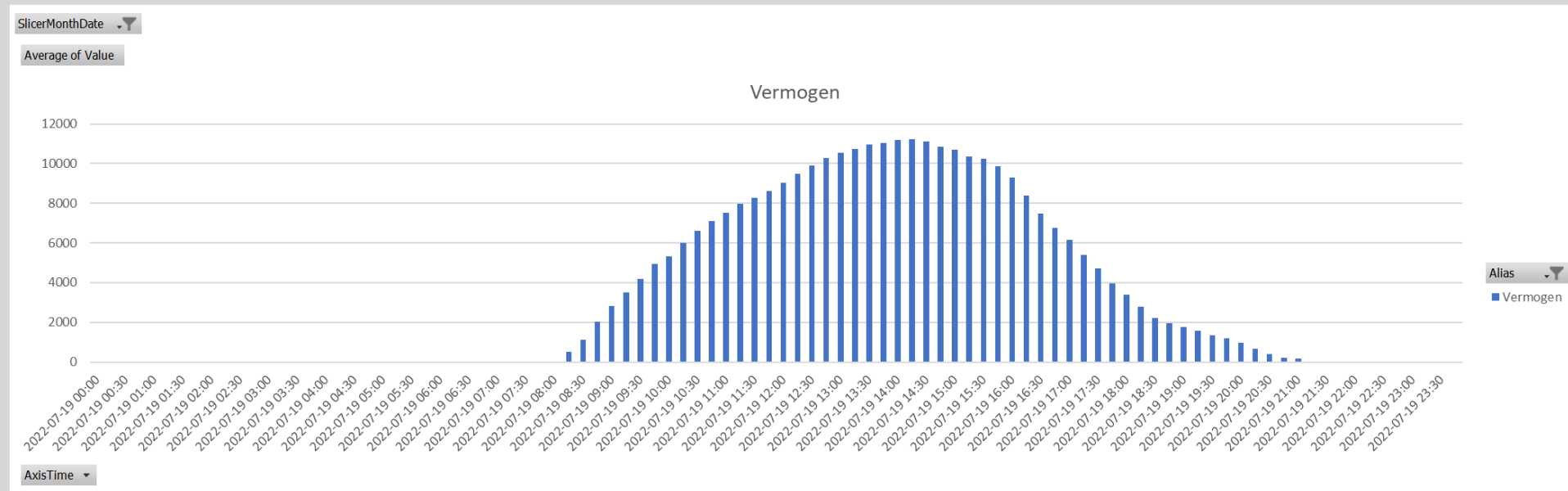
Figuur 1: vermogen gemeten op 19-juli-2022 in Watt
